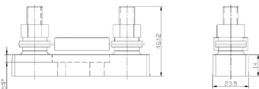
MEGA-Sicherung
