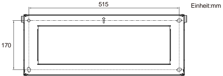
Abbildung 4.23 - Wandmontage des Wechselrichters
