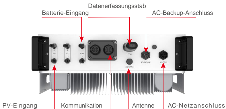
Abbildung 1.12 - Seitenansicht von unten
