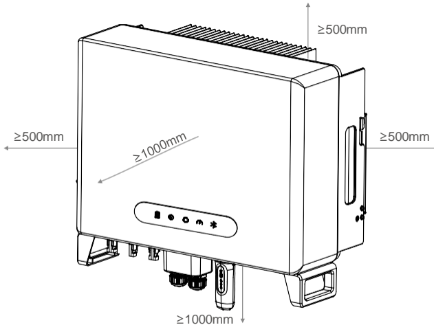
Abbildung 4.12 - Montageabstand des Wechselrichters
