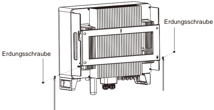
Abbildung 4.5 Anschluss des externen Erdungsleiters
